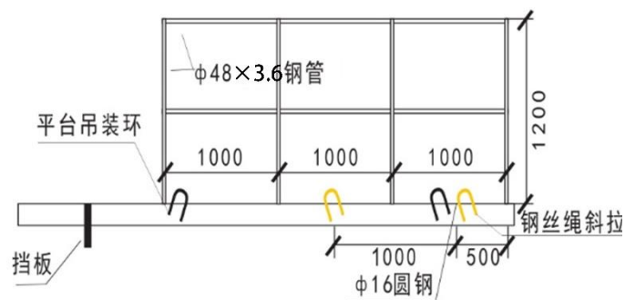
侧立面图
