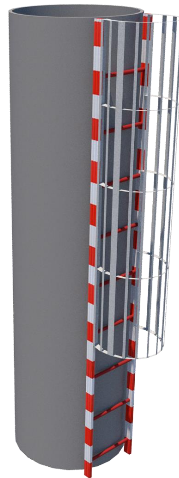
钢柱登高挂梯构造图
