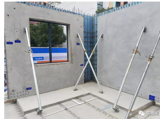
预制剪力墙临时支撑
