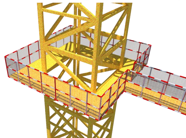
钢管搭设式操作平台示意图
