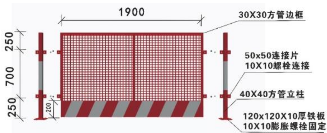
栏杆构造设计图（一）
