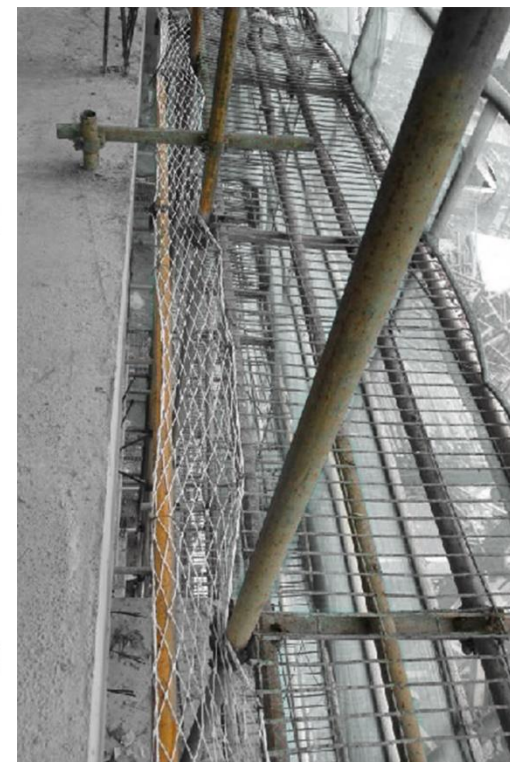
安全兜网防护
