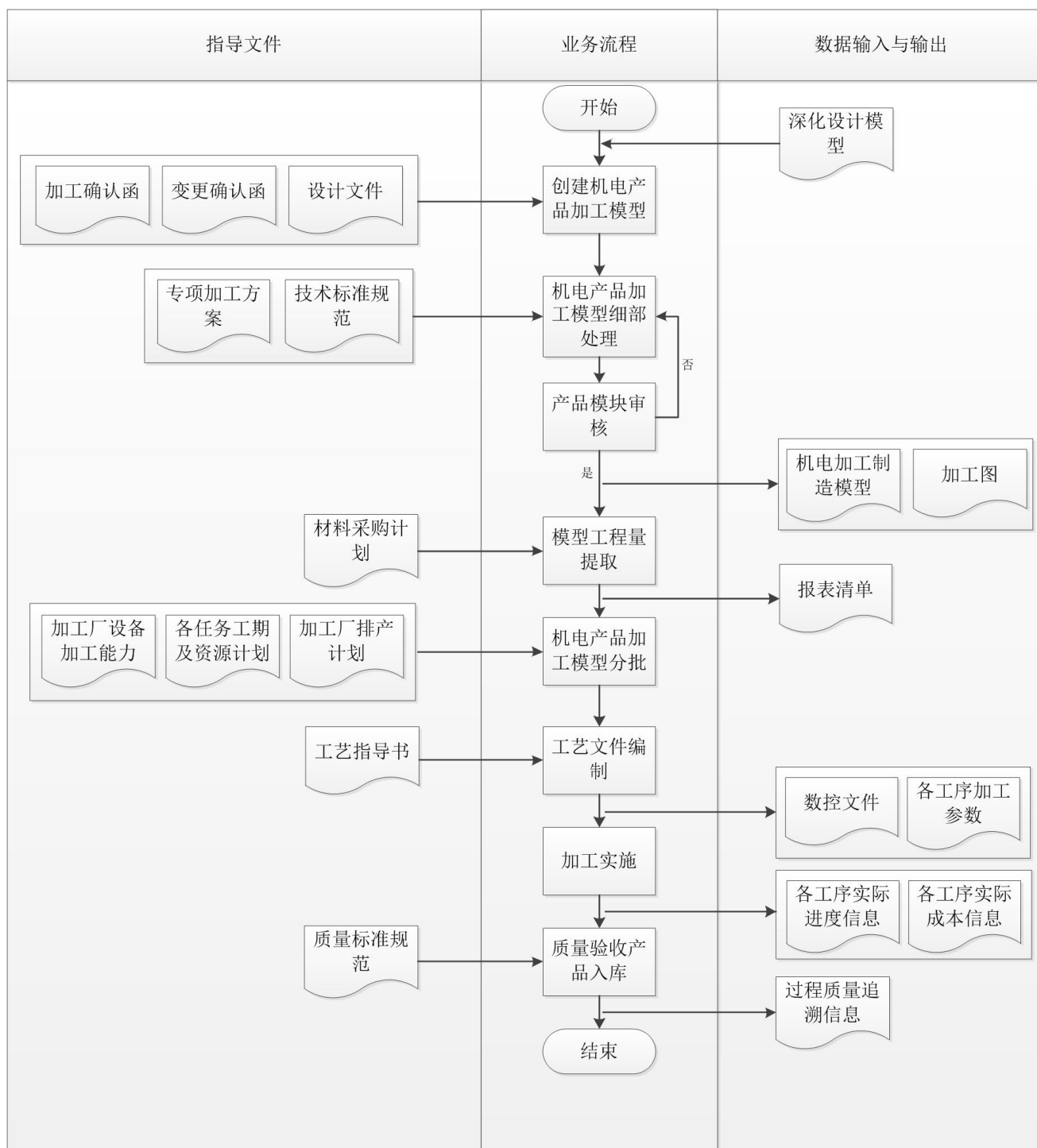
图 7.4.2 机电产品加工 BIM 典型应用示意图
