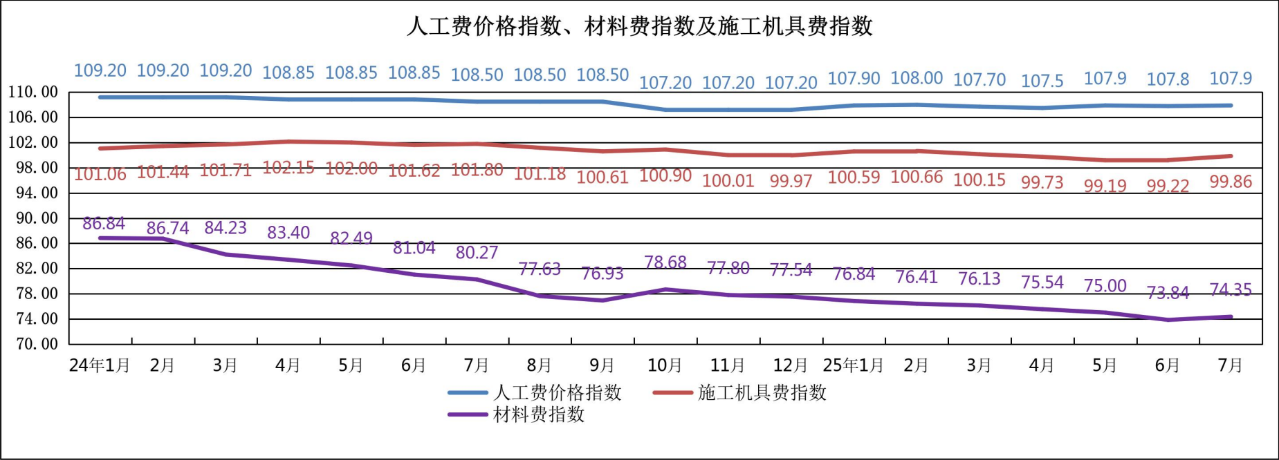
2025 年 7 月广州市市政工程人工费价格指数、材料费指数及施工机具费指数走势图
