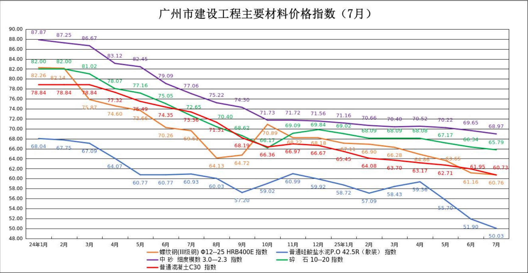
2025 年 7 月广州市建设工程主要材料价格指数走势图
