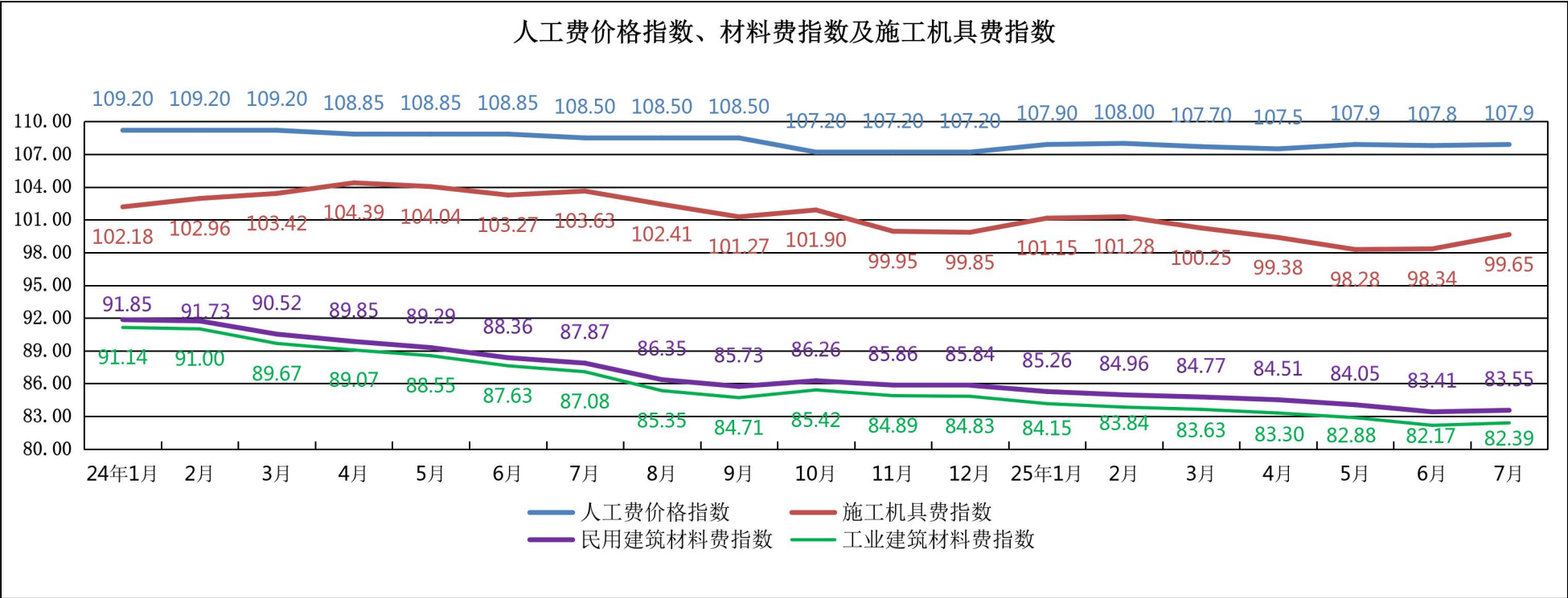
2025 年 7 月广州市房屋建筑人工费价格指数、材料费指数及施工机具费指数走势图
