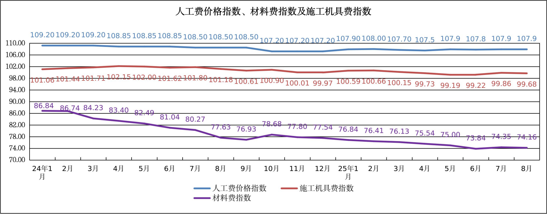
2025 年 8 月广州市市政工程人工费价格指数、材料费指数及施工机具费指数走势图
