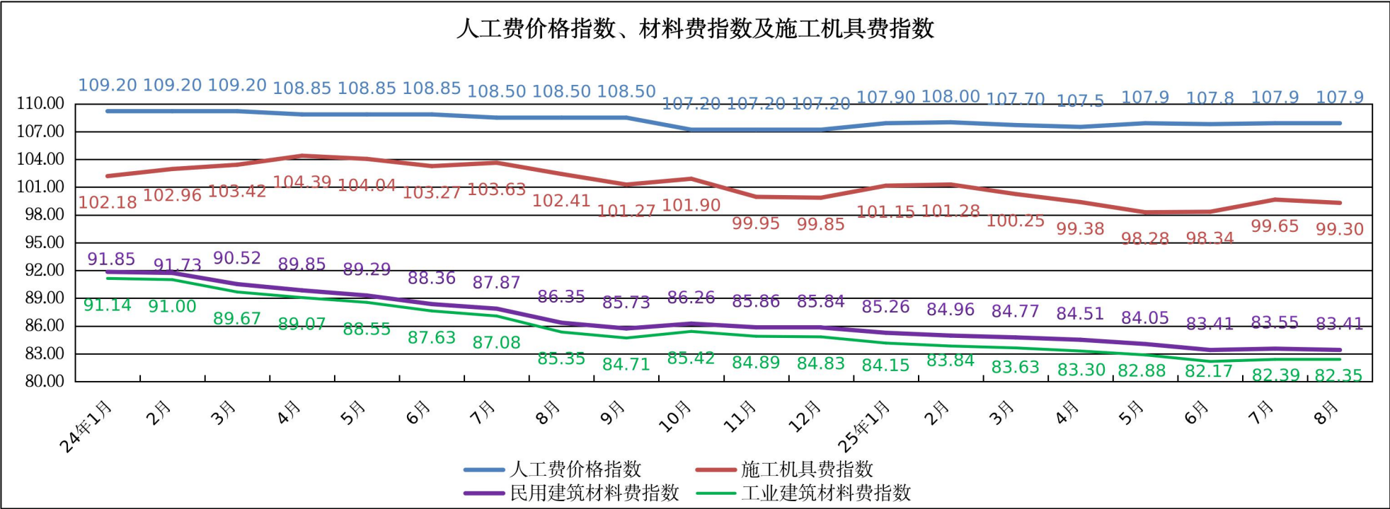
2025 年 8 月广州市房屋建筑人工费价格指数、材料费指数及施工机具费指数走势图
