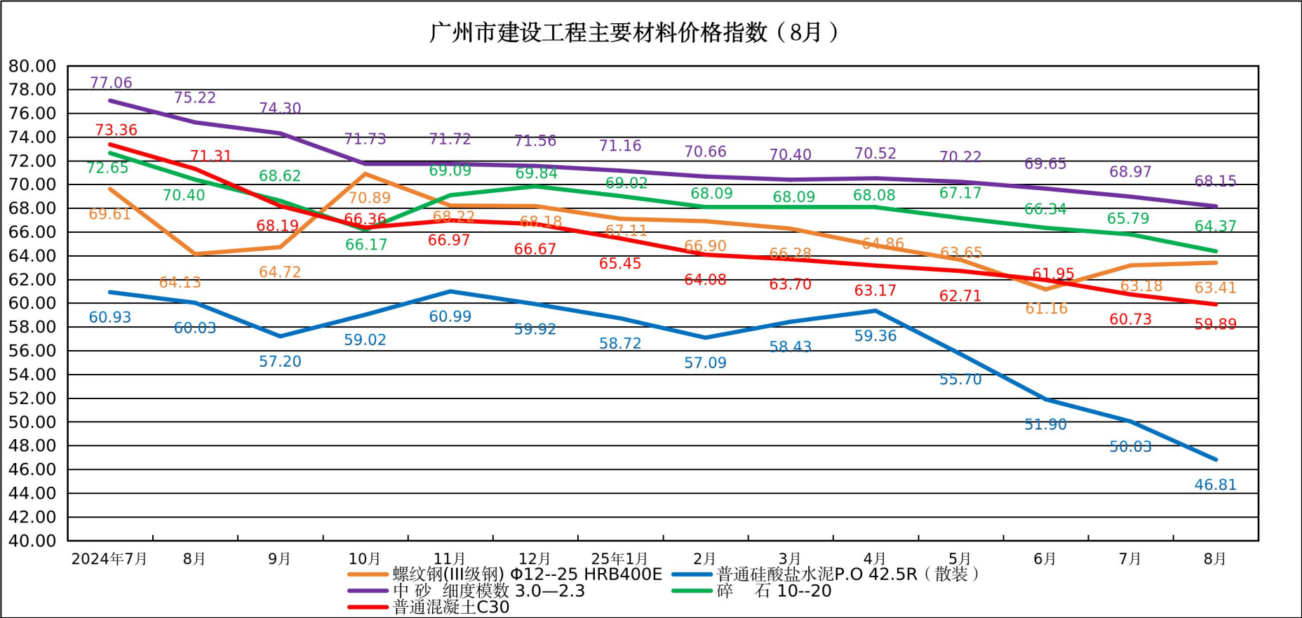
2025 年 8 月广州市建设工程主要材料价格指数走势图
