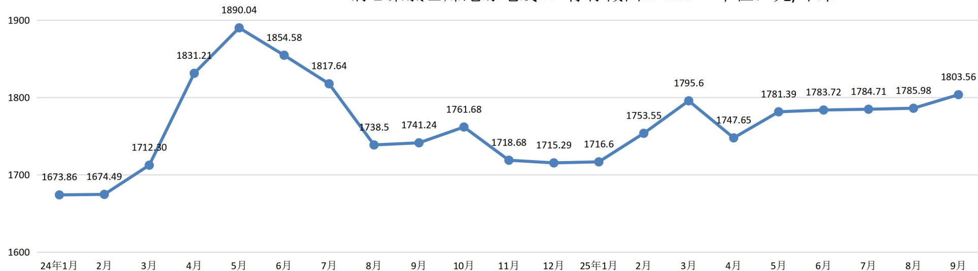
铜芯聚氯乙烯绝缘电线BV 标称截面2.5mm 2 单位：元/千米
