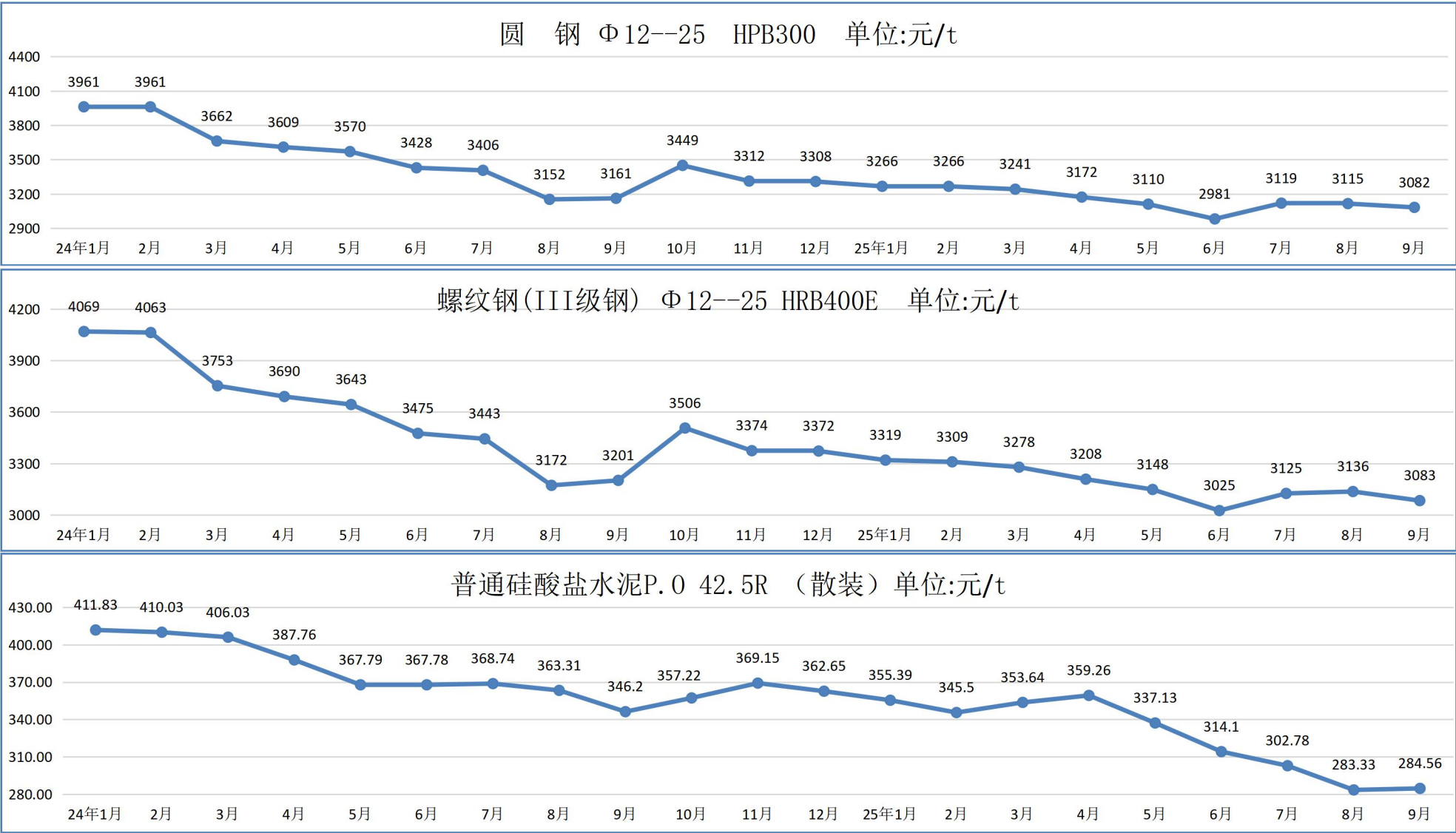
2025 年 9 月广州市建设工程 22 种常用材料税前综合价格走势图
