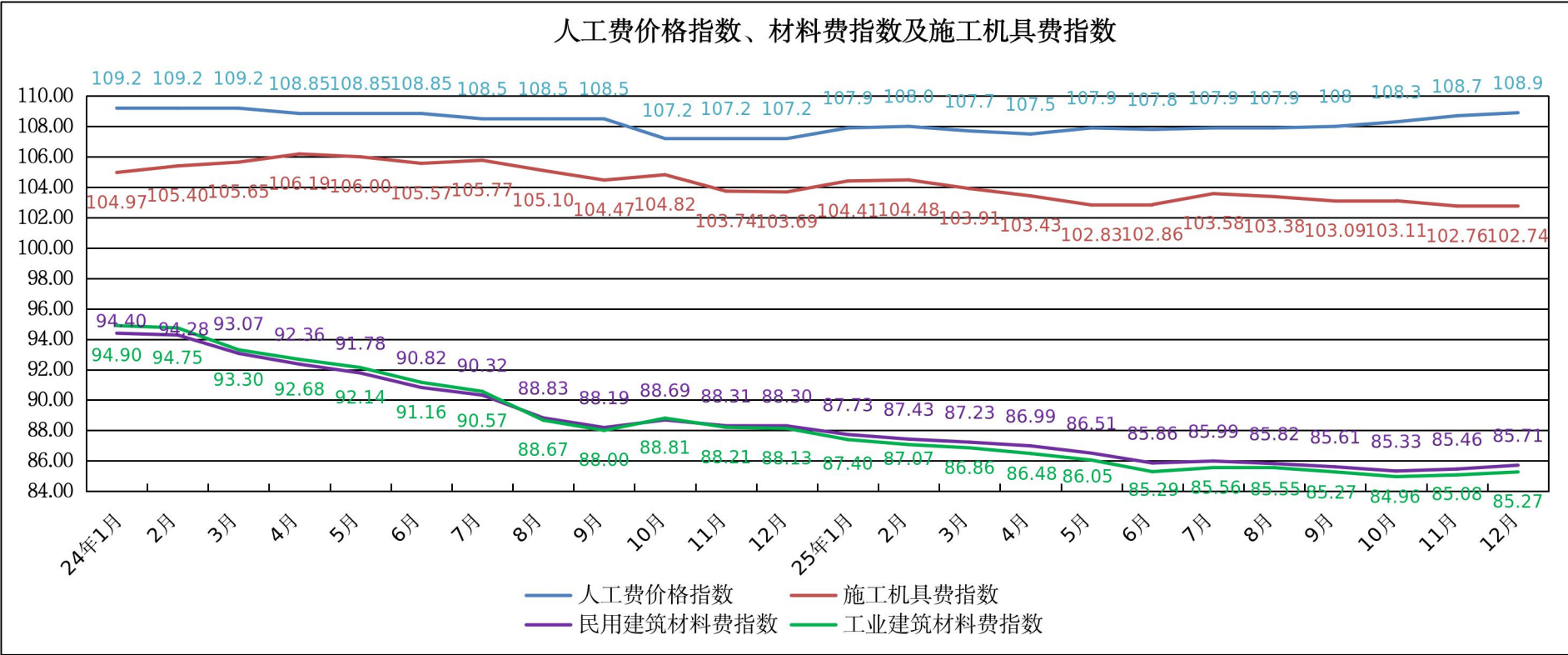
2025 年 12 月广州市房屋建筑工程人工费价格指数、材料费指数及施工机具费指数走势图
