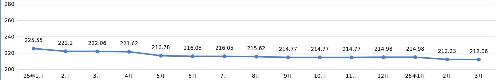
蒸压加气混凝土砌块 B07 A5.0 合格品 单位:元/m 3
