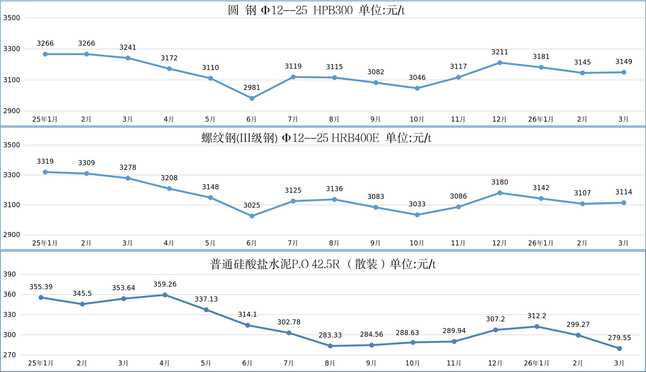
2026 年 3 月广州市建设工程 22 种常用材料税前综合价格走势图
