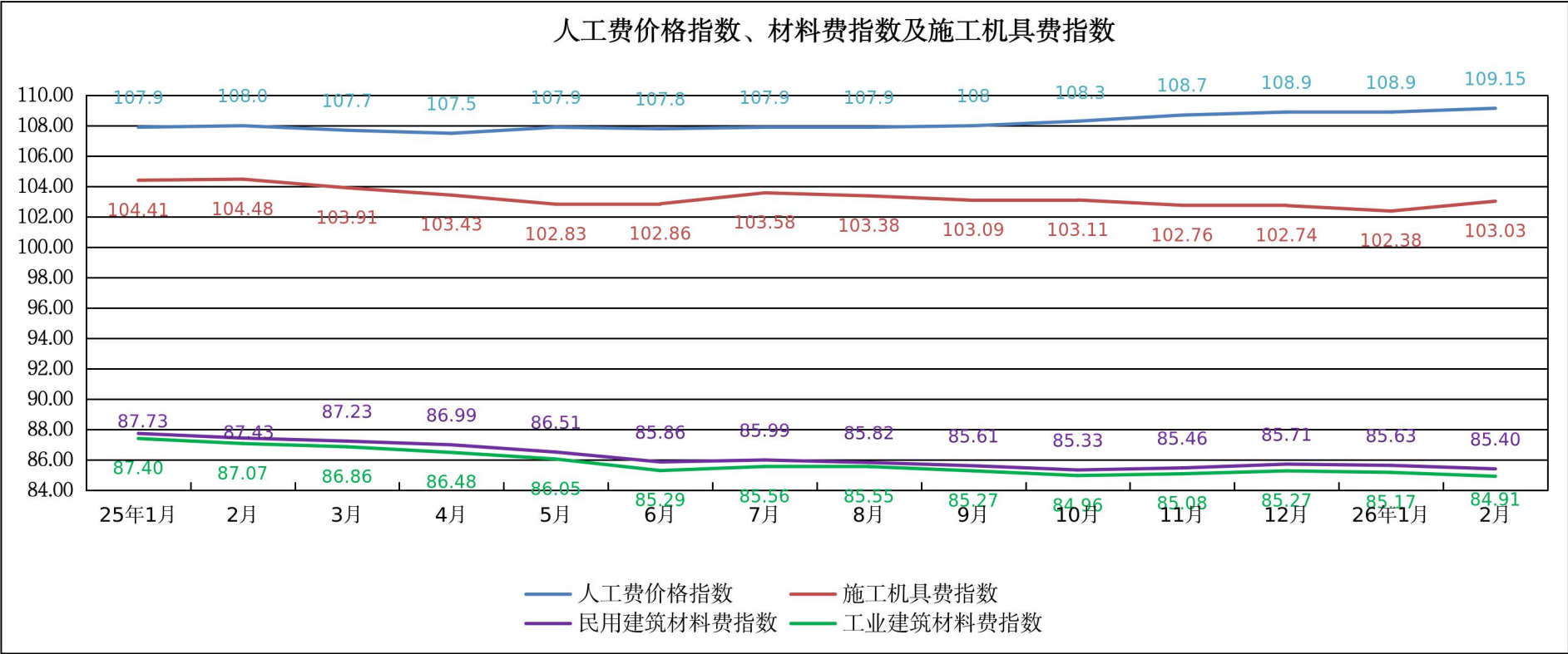
2026 年 3 月广州市房屋建筑工程人工费价格指数、材料费指数及施工机具费指数走势图
