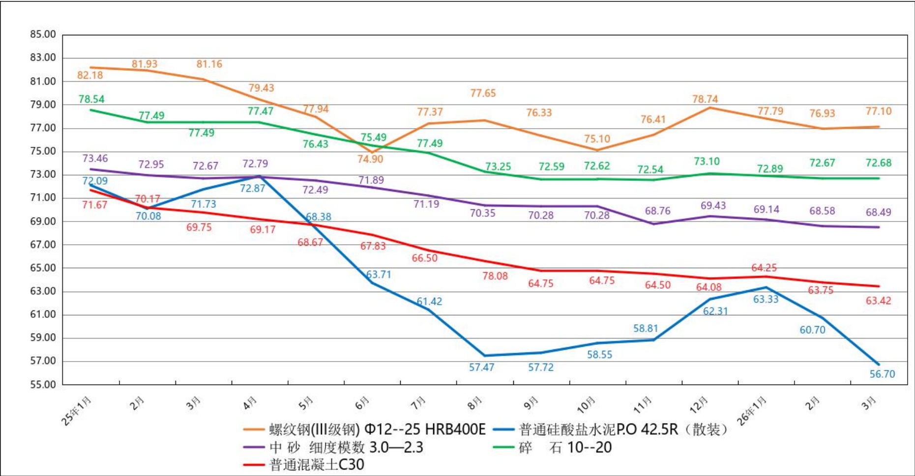
2026 年 3 月广州市建设工程主要材料价格指数走势图
