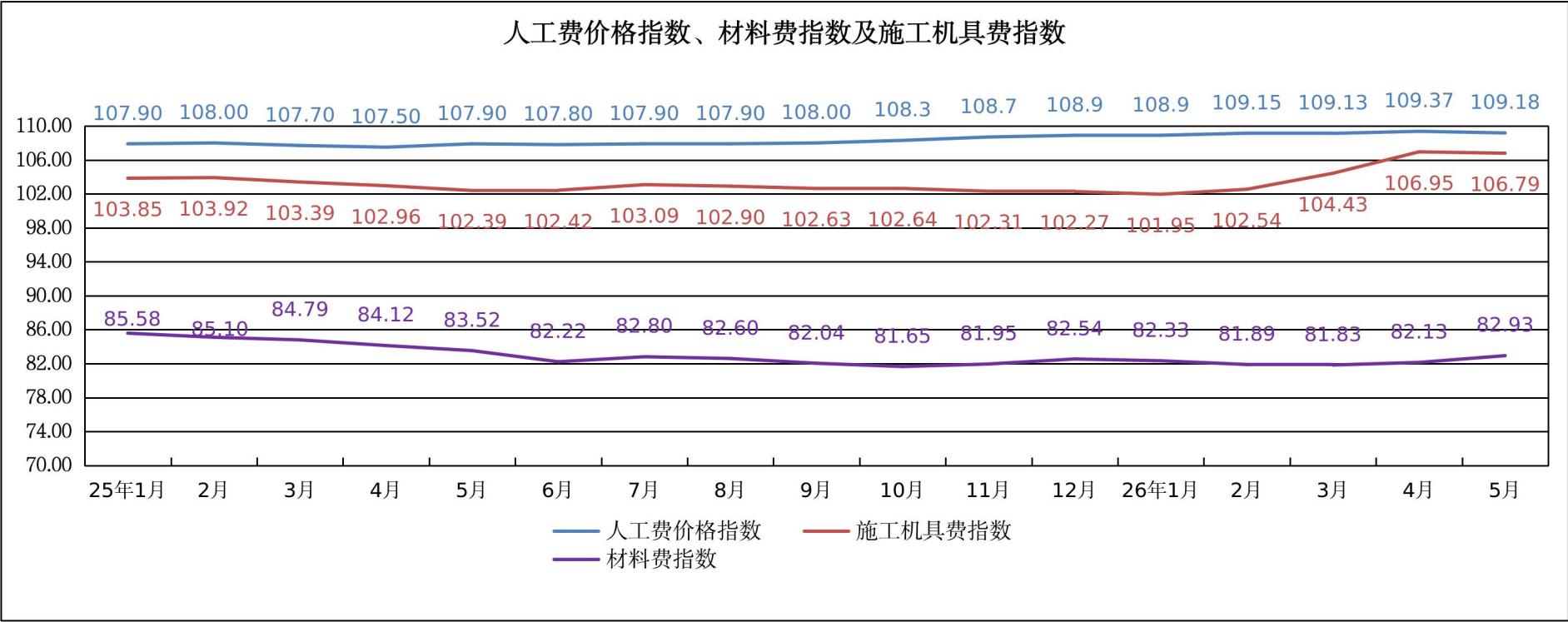
2026 年 5 月广州市市政基础设施工程人工费价格指数、材料费指数及施工机具费价格指数走势图
