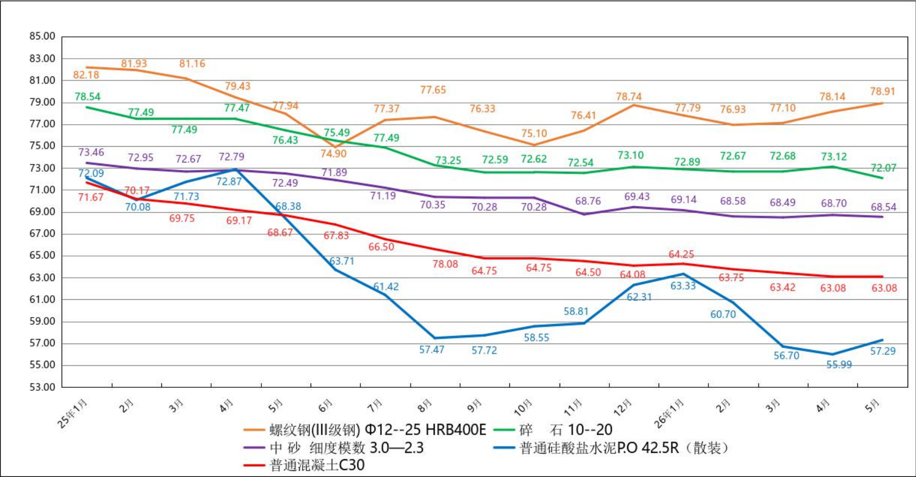
2026 年 5 月广州市建设工程主要材料价格指数走势图
